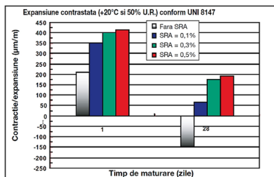
FIG. 2 - Valori obtinute cu mortare continand ciment CEM I 52,5 R, nisip normalizat si apa, conform compozitiei indicate in Standardul EN 196-1, si 7% aditiv Expancrete
