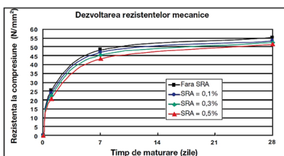
FIG. 3 - Valori obtinute cu mortare continand ciment CEM I 52,5 R, nisip normalizat si apa, conform compozitiei indicate in Standardul EN 196-1
