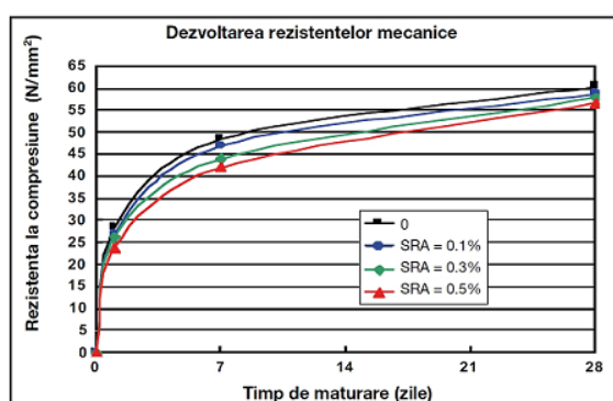
FIG. 4 - Valori obtinute cu mortare continand ciment CEM I 52,5 R, nisip normalizat si apa, conform compozitiei indicate in Standardul EN 196-1, si 7% aditiv Expancrete
